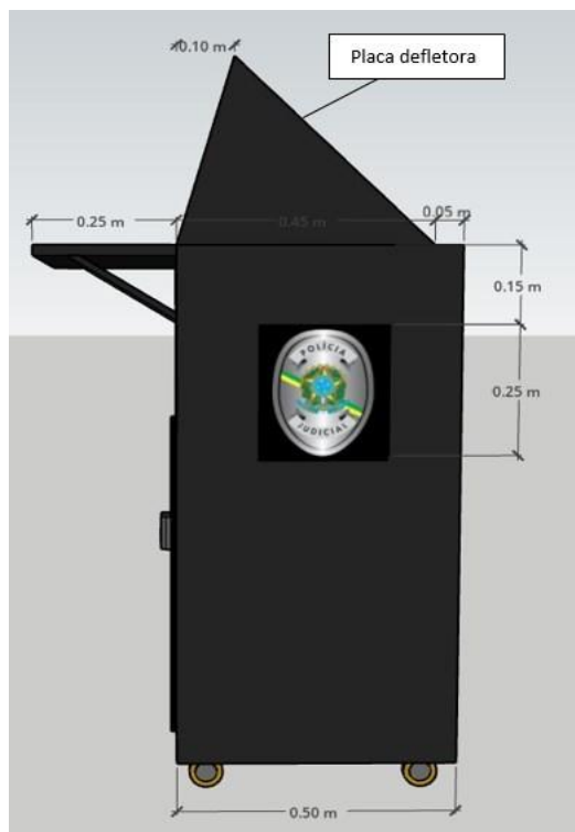
Figura 2 - Vista lateral
