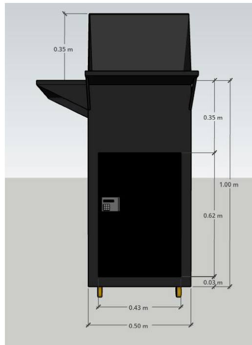
Figura 1 – Vista frontal
