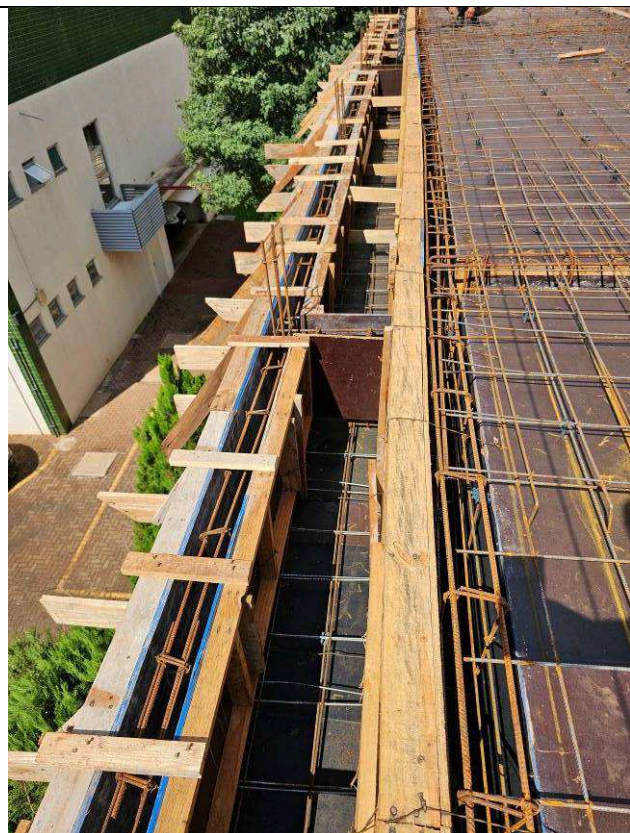
Figura 15: Formas e armaduras - cobertura.
