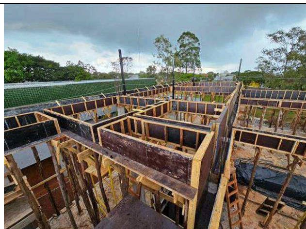
Figura 10: Montagem das formas.
