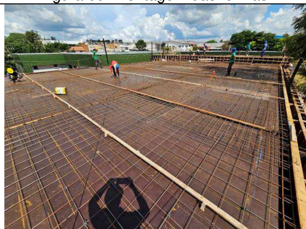
Figura 11: Formas e armaduras - cobertura.
