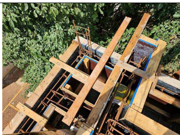
Figura 14: Formas e armaduras - cobertura.
