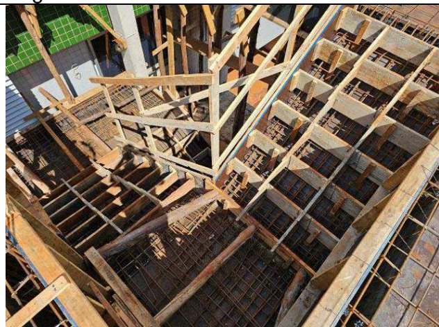
Figura 22: Formas e armaduras - escada.
