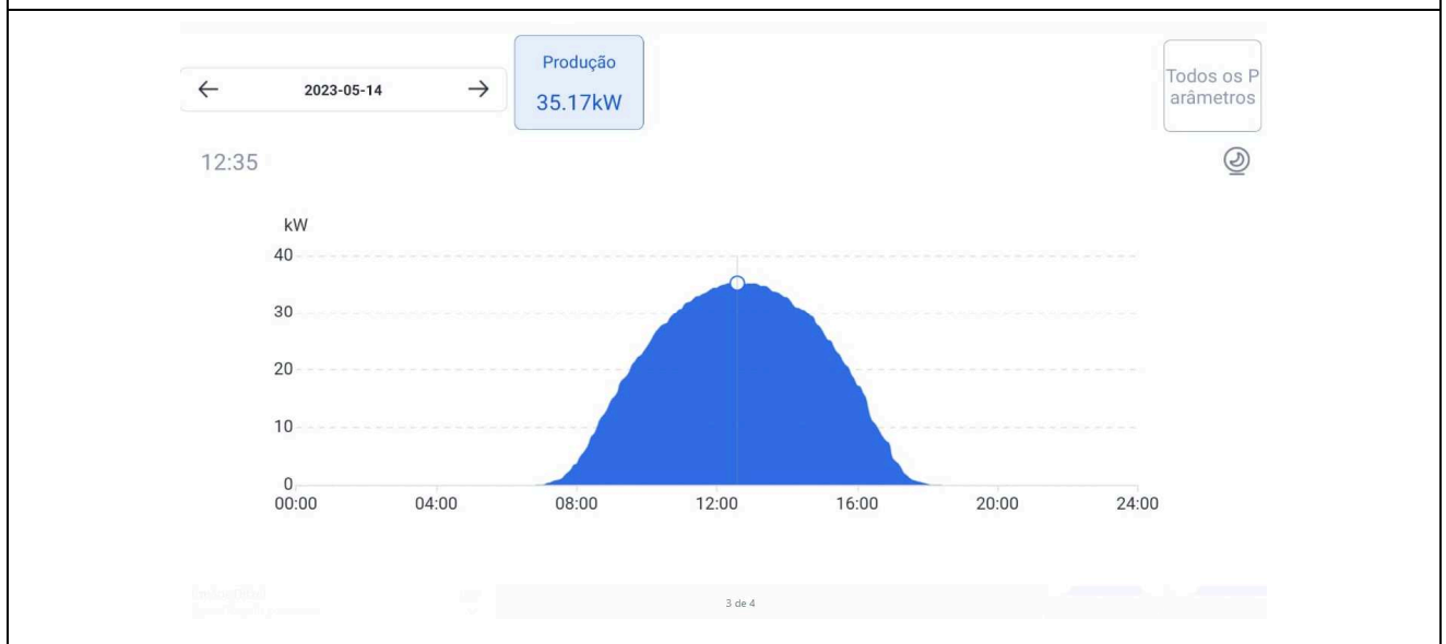
Figura 02 – Gráfico de geração do dia 14/05/23 (aplicativo Solarman) - Toledo
