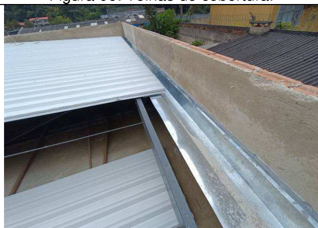
Figura 08: Telhas de cobertura.
