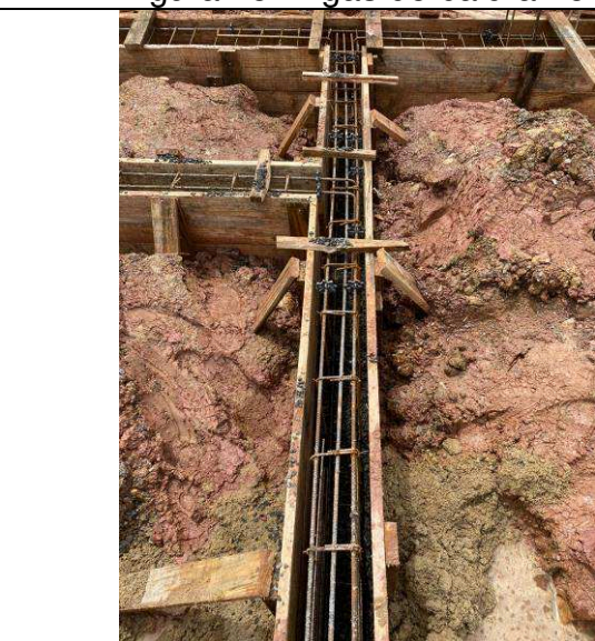
Figura 27: Vigas de baldrame.
