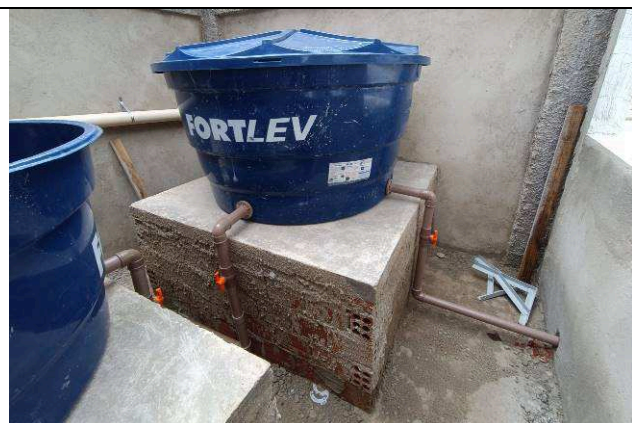
Figura 11: Reservatório de água potável, registros e tubulações de distribuição.
