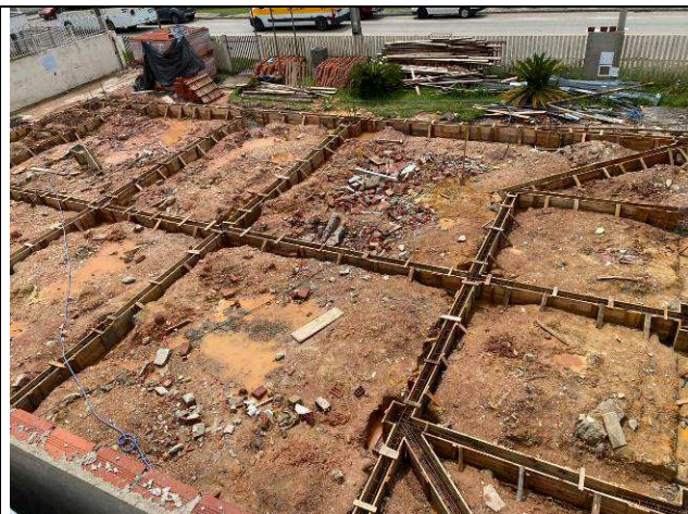
Figura 29: Vigas de baldrame montadas.
