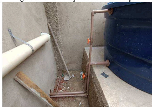
Figura 14: Tubulação de alimentação.
