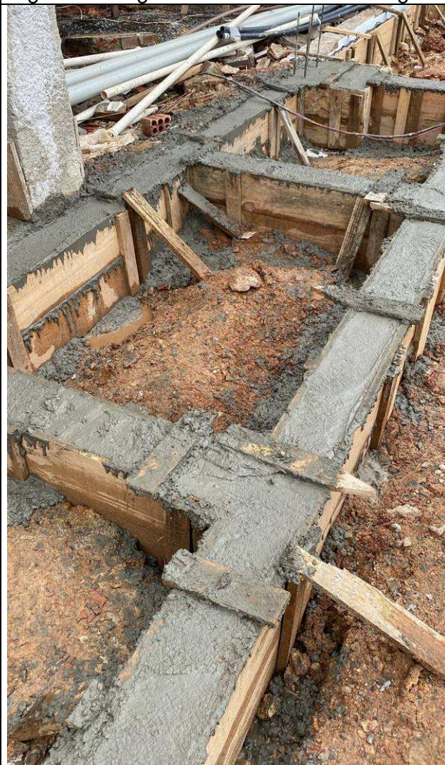
Figura 32: Vigas de baldrame concretadas.
