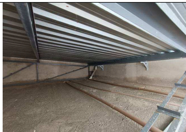
Figura 09: Telhas de cobertura e tubulações de água fria.
