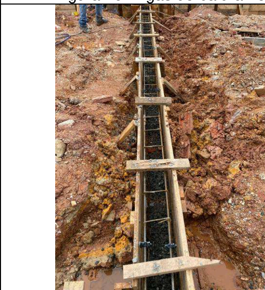
Figura 28: Vigas de baldrame.
