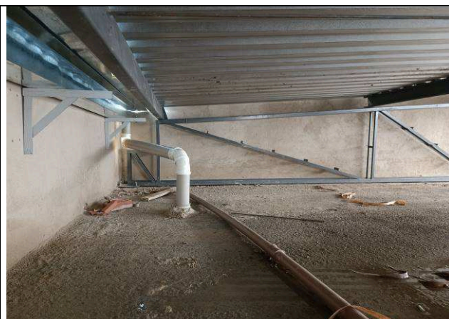
Figura 10: Telhas de cobertura e tubulações de água fria.
