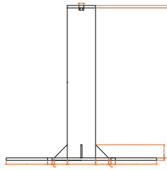
ELEVAÇÃO FRONTAL ESC: 1/50
