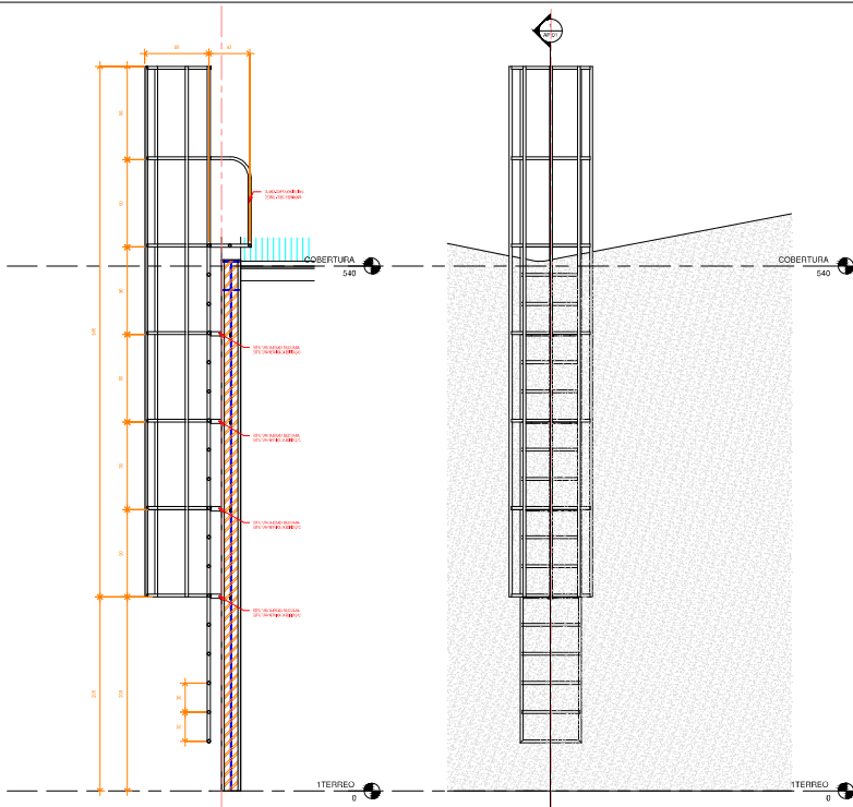
1 Corte Longitudinal AP 01 1 : 20
