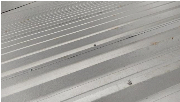
Figura 05C: Detalhe da fixação das telhas às terças
