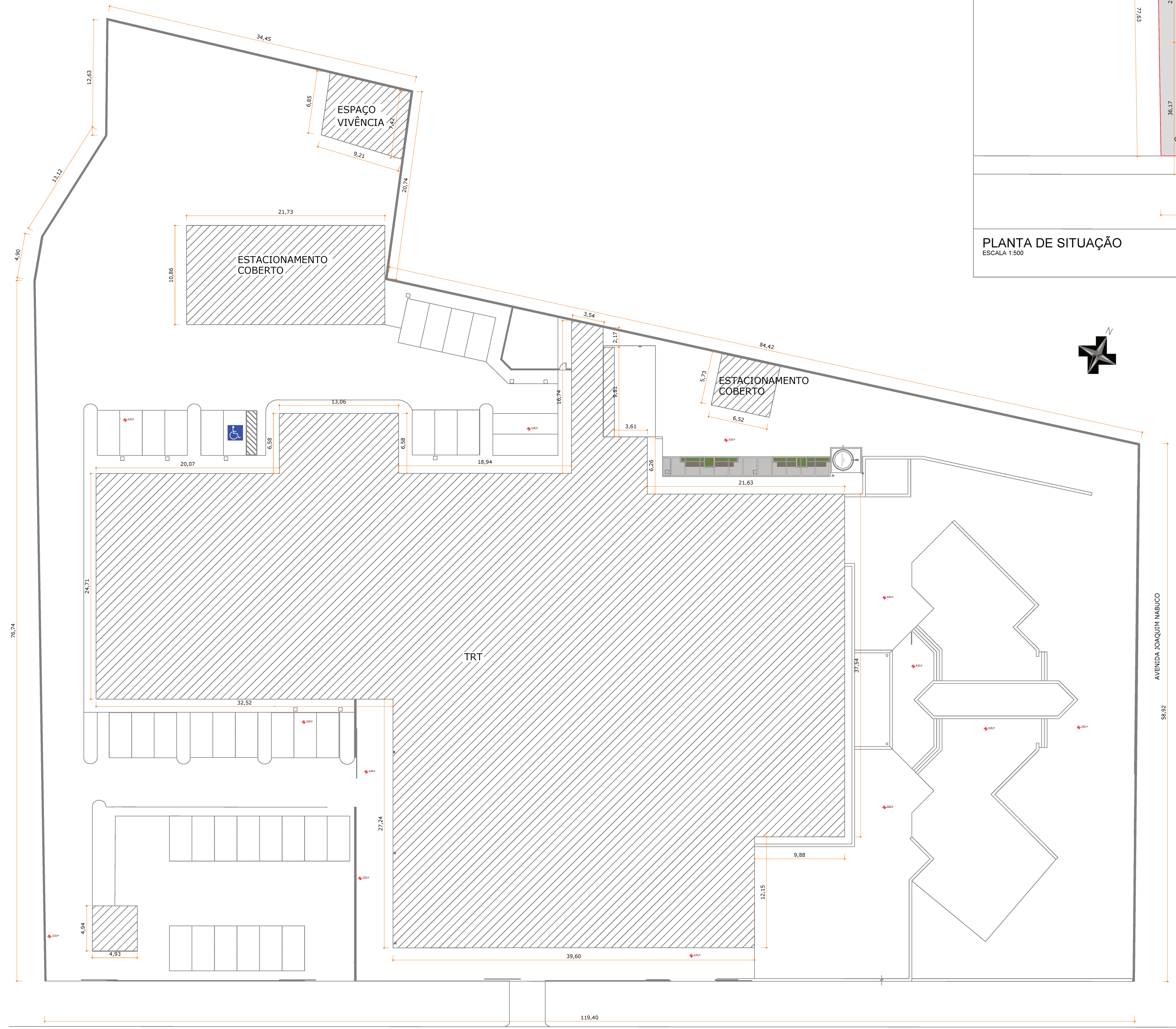
PLANTA DE IMPLANTAÇÃO ESCALA 1:200
