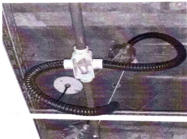
Figura 05: Eletroduto flexível metálico
