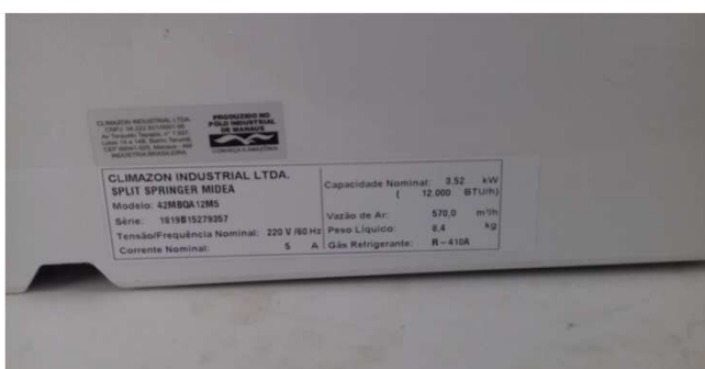
Figura 12C: Decalque de evaporadora - sala técnica
