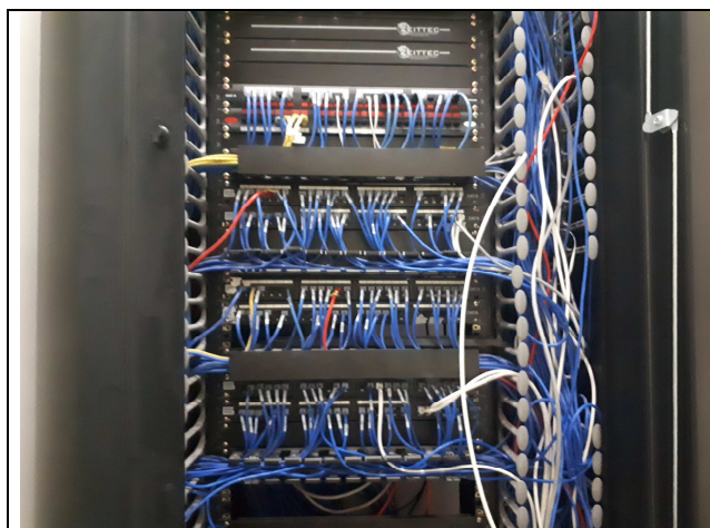
Figura 5E - rack 1º pavimento
