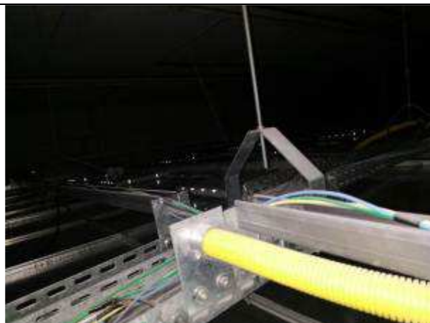
Figura 03E - Infraestrutura e cabeamento elétrico
