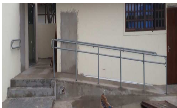
Figura 12 - Execução de alvenaria, aterro, lastro de concreto, armação, grelha e tubo de drenagem. O Corrimão deve ser corrigido.
