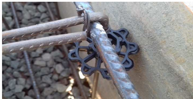
Figura 8: Detalhe de ferragem e espaçador
