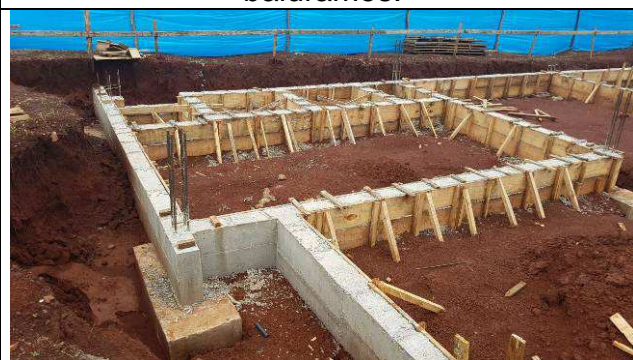
Figura 42C: Vigas baldrames concretadas.
