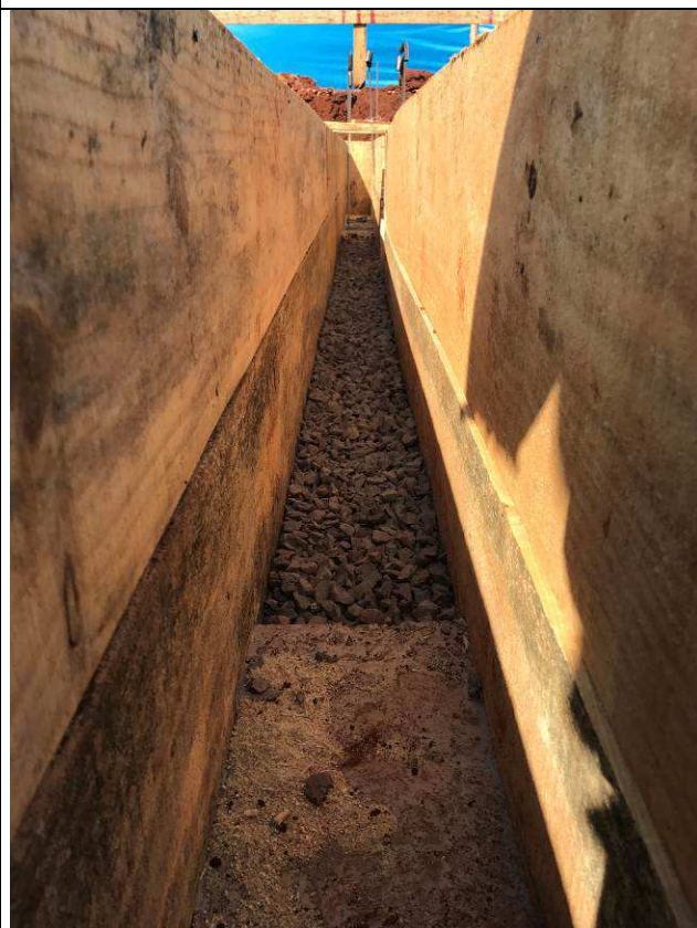
Figura 18C: Montagem das formas das baldrames e lastro de obra.
