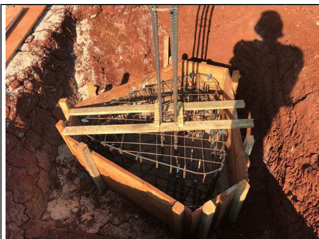
Figura 07C: Formas e armaduras - P07.
