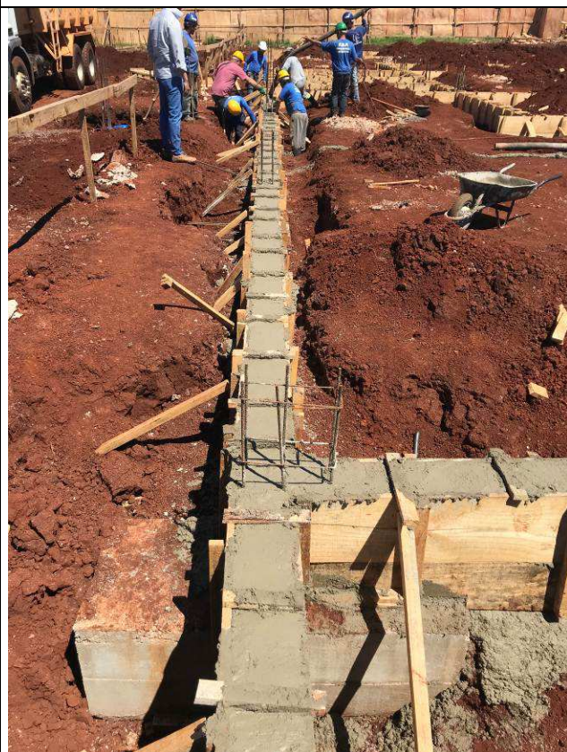
Figura 32C: Concretagem das vigas baldrames.
