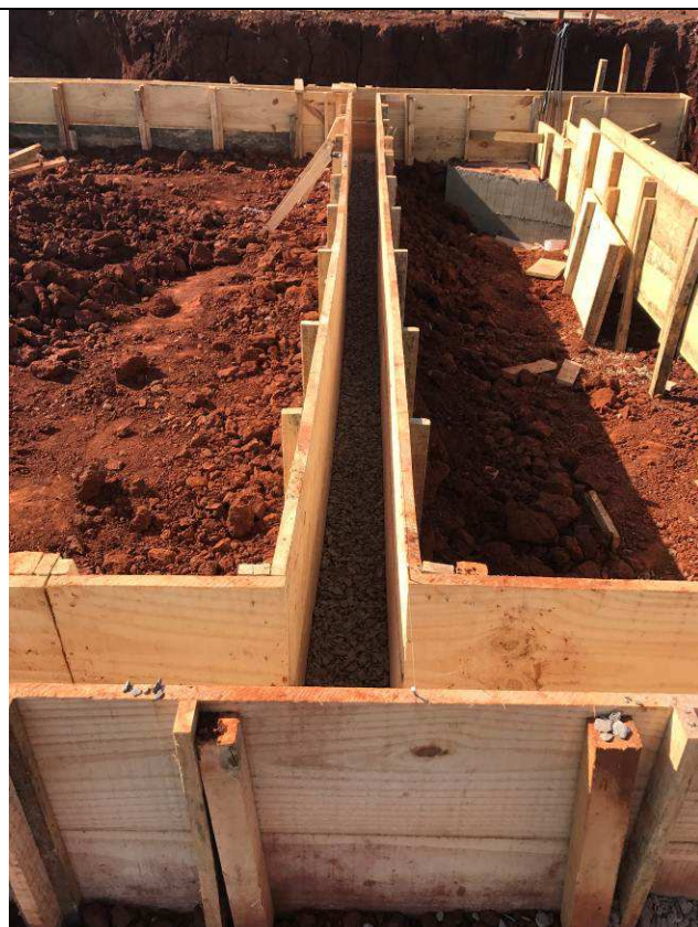
Figura 17C: Montagem das formas das baldrames e lastro de obra.
