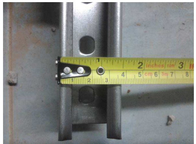
Figura 08E: Aferição de dimensão do perfilado #38x38
