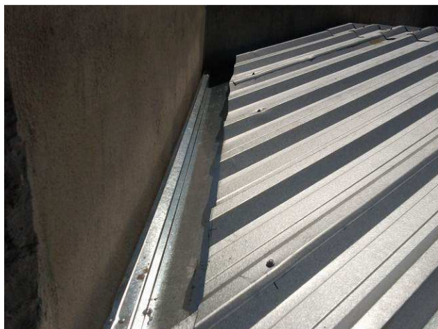
Figura 13C: Calhas instaladas Curitiba, 23 de outubro de 2014.
